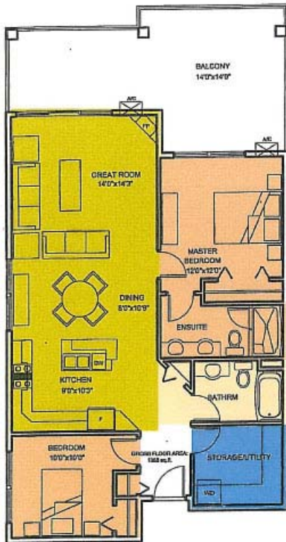
SUITE 203,303 (TYPE6)
