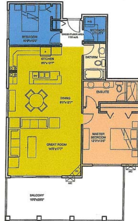
SUITE 204,304 (TYPE7)
